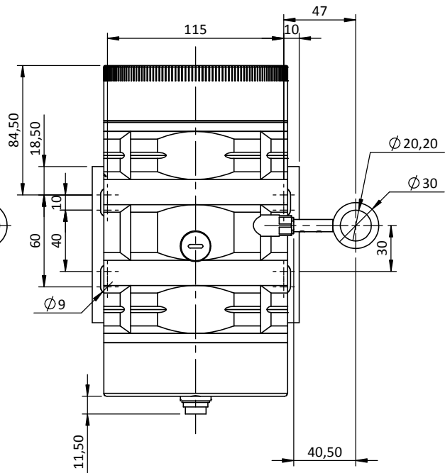
C connection (Connector M16 - DIN 3 pin)
